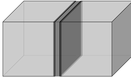
Fig. 6. \Omega^{m,\epsilon}
