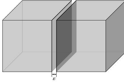
Fig. 4. \Omega^{out,\epsilon} = \Omega^{+,\epsilon} \cup \Omega^{-,\epsilon}
