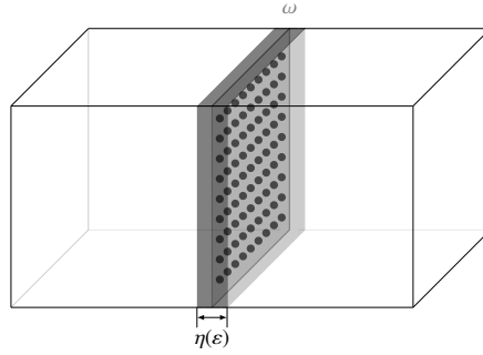
Fig. 5. \Omega^{in,\epsilon}
