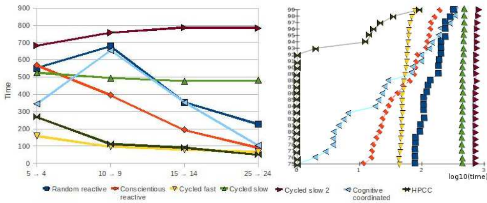
FIGURE 3: temps de stabilisation (gauche), courbes de stabilisation pour le scénario 15 → 14 (droite)
