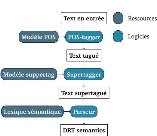
FIGURE 1 – Schéma des ressources et outils de la chaîne de traitement
