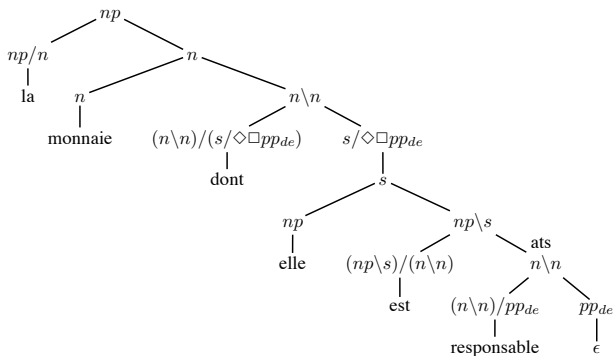
FIGURE 4 – résultat de l'extraction
