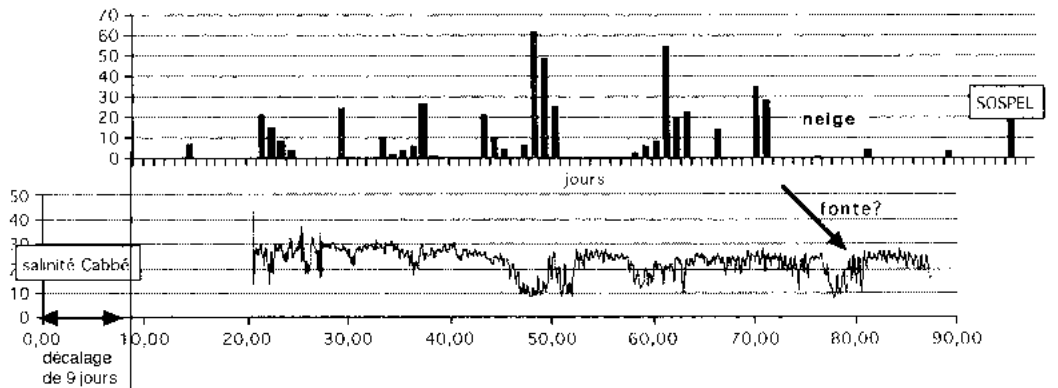
Figure 6. Essai de corrélation entre les variations de salinité de la source de Cabbé-Massolins et les données pluviométriques du moyen-pays niçois. Secteurs de Peille (col de la Madone) et de Sospel.
