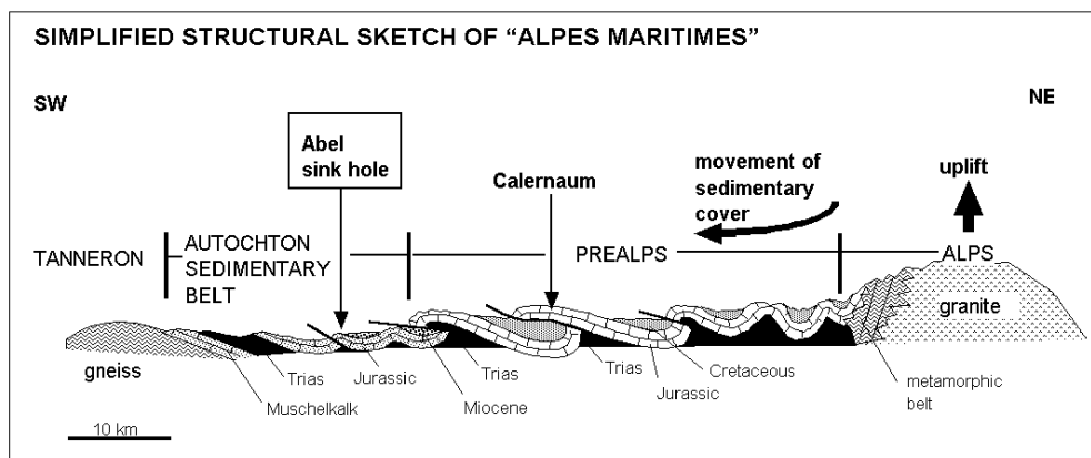
Figure 3: Simplified structural sketch of Alpes Maritimes between Mercantour and Tanneron. Schéma structural simplifié des Alpes Maritimes entre le Mercantour et le Tanneron.
