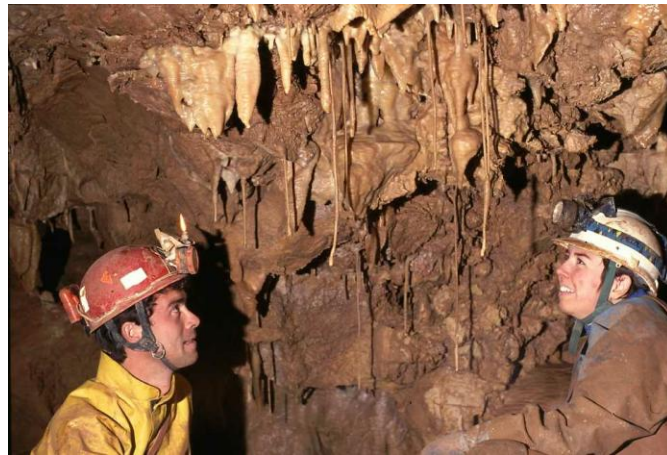
Figure 8: Curved sodastraws under a rock that rotates under the thrust fault plane. Fistuleuses courbées sous un bloc en rotation sous le plan de chevauchement de l'Aven Abel.
