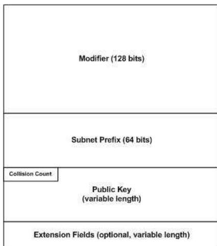
Fig. 4. CGA Parameters
