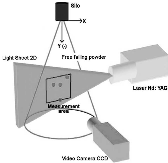
Fig. 4. PIV system.
