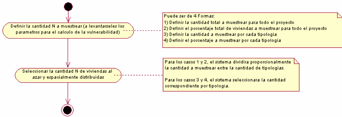
Figura 143. Diagrama de actividad para el Caso de Uso: SeleccionarMuestras
