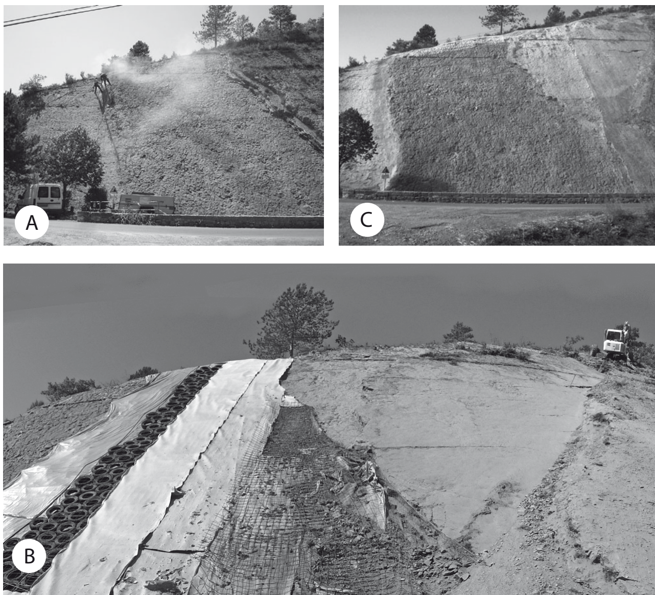
Fig. 5: Le chantier de sécurisation, de conservation et de mise en valeur de la «Dalle» en 2009. A. Le début du chantier en 2009 (Photo M. GUIOMAR). B. Vue panoramique du chantier (photo J. BOURIDEYS). Sur la gauche, des protections recouvrent les ammonites et sur la droite une pelle-araignée effectue le déroctage des surplombs. C. Le site de la «Dalle à ammonites» à l'issue du chantier de 2009.
