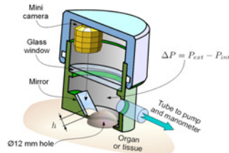
Figure 1. Vue en coupe de LASTIC : la partie supérieure contient la caméra tandis que la chambre d'aspiration et le miroir sont dessous (gauche). Modules de Young déterminés par LASTIC et les machines de traction pour chaque matériau (droite).
