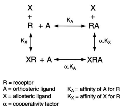
Fig. 4. Modèle du complexe ternaire (Birdsall et al. , 2005).
