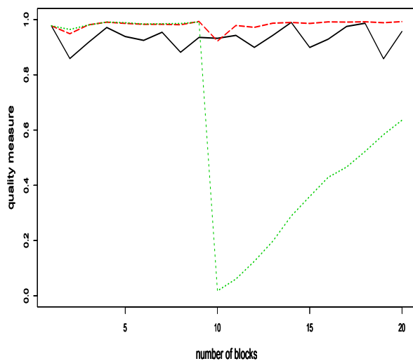
Figure 1: Comportement numérique des estimateurs de SIRds, SIRu et SIR. L'image à gauche représente la qualité \cos^2(\hat{\beta}_t, \beta_t) , en fonction du nombre de blocs (en tirets rouges pour SIRdatastream, en pointillés vert pour SIRu, en noir pour SIR sur uniquement le bloc t ). L'image à droite représente les poids \cos^2(\hat{b}_t, \hat{b}_T) utilisés dans le calcul de \widehat{M}_T .
