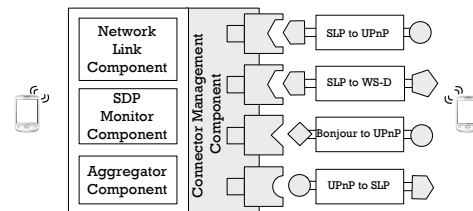
Fig. 2. ZigZag Middleware
