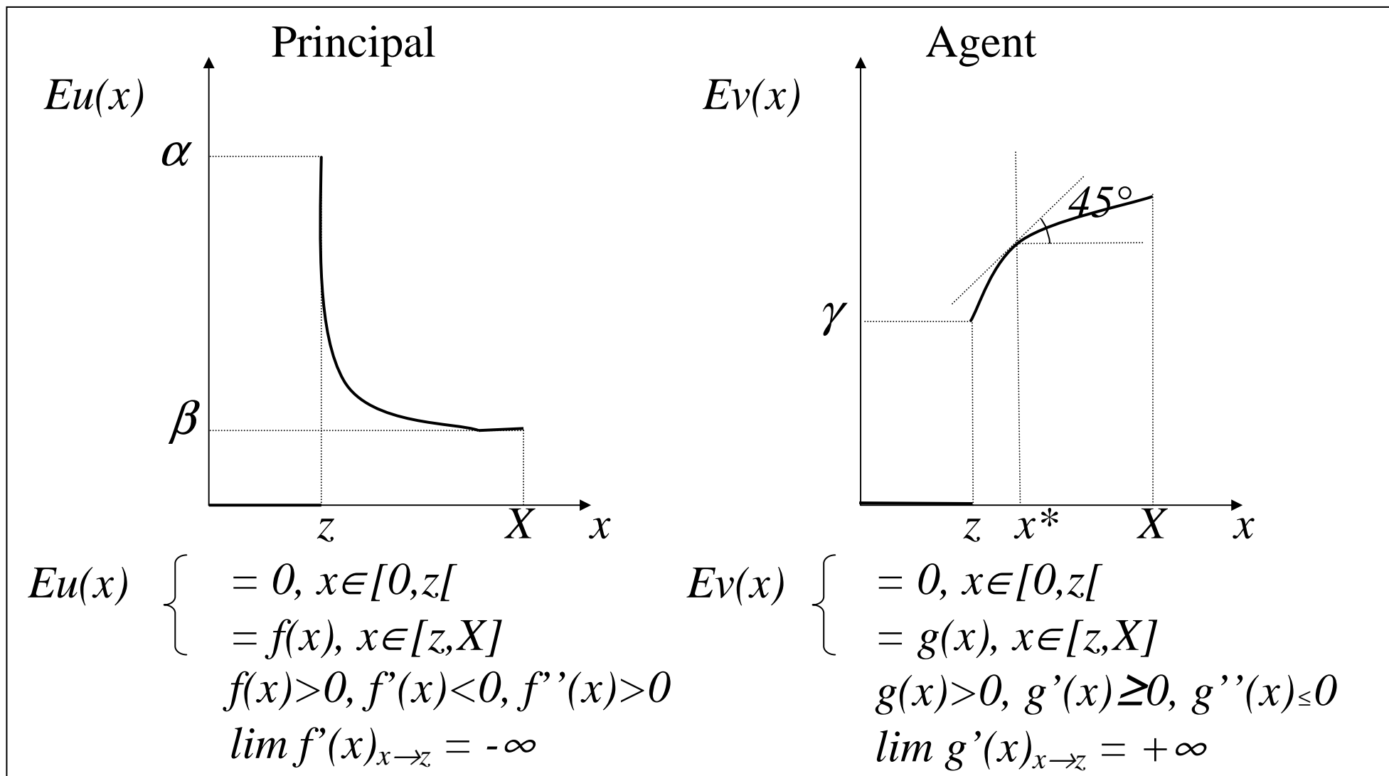
Figure 4 Jeu de faux semblants de moyen terme,
