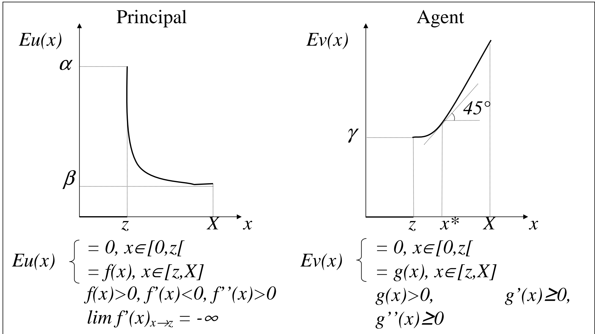
Figure 1 Jeu de faux semblant de moyen terme, version "forte" : cas b > 1
