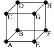
\mathcal{K}_0
