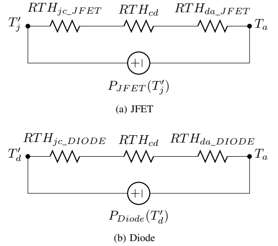
FIGURE 9: Modèle thermique
