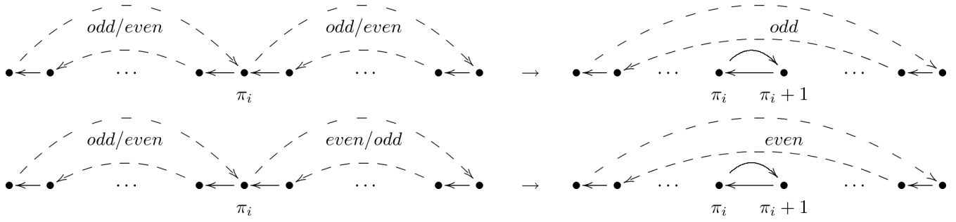
Fig. 8. Proof of Lemma 7.2
