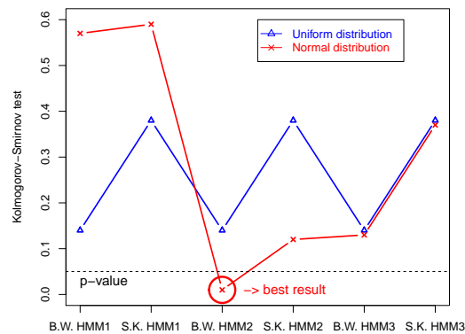
(b) Kolmogorov-Smirnov test statistic
