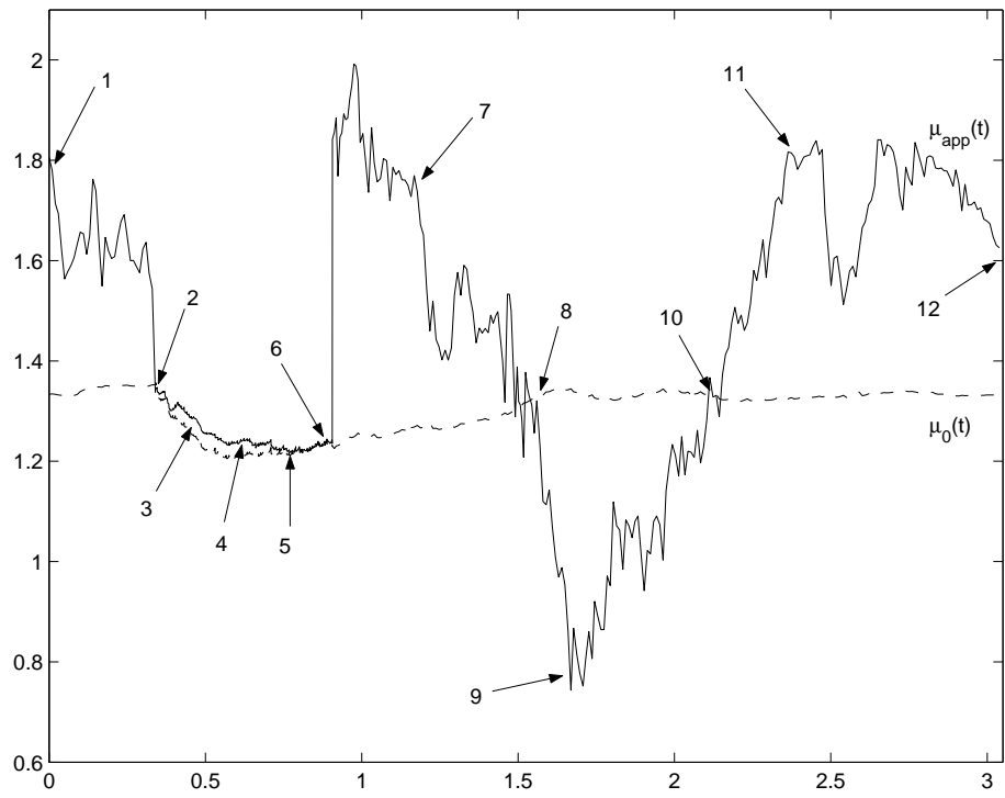
Figure 6 : Apparent viscosity versus time. Viscosité apparente en fonction du temps.
