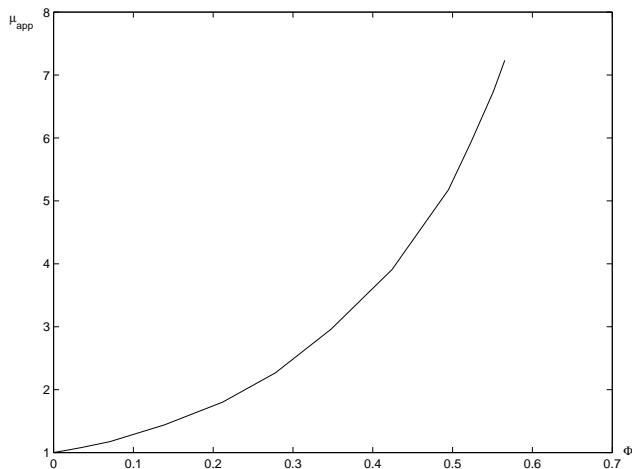
Figure 4 : Apparent viscosity with respect to solid fraction for uniform distributions. Viscosité apparente en fonction de la fraction solide pour une distribution uniforme.
