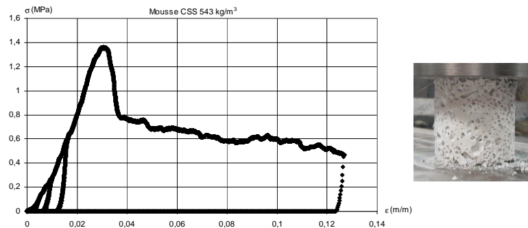
Figure 6. Essai de compression : courbe contrainte vs déformation
