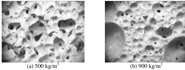
Figure 3. Connectivité des alvéoles pour deux densités de mousse différentes (base de la photo = 5 mm).
