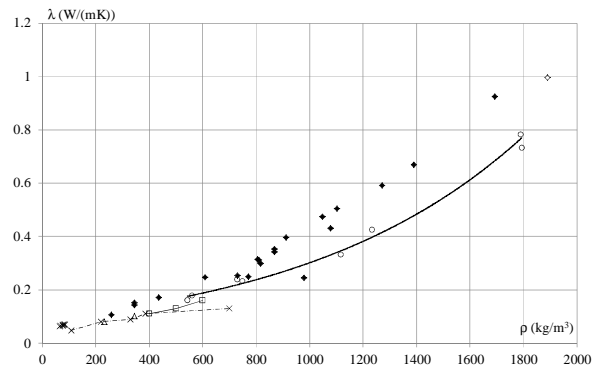
Figure 5. Evolution de la conductivité thermique vs la masse volumique : rond : mousses CSS, losange : Mousses de gypse, croix : béton de chanvre et paille, carré : béton cellulaire, triangle : béton de polystyrène.
