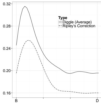
(d) \sqrt{\text{Var}(\hat{f}), n = 1000}
