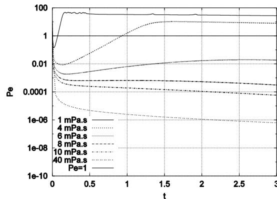
Figure 4 : Pe=f(t) pour Bi=0,2 et différentes viscosités de la solution
