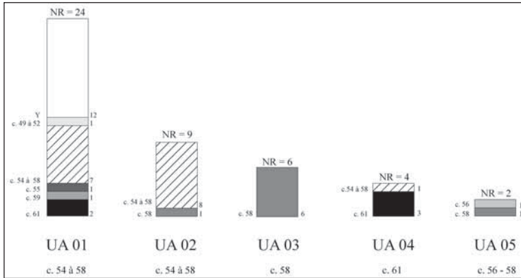
Figure 165 - Schéma de dispersion verticale des 5 unités d'appariements reconnues. NR = nombre de restes. UA = Unité d'appariements.
