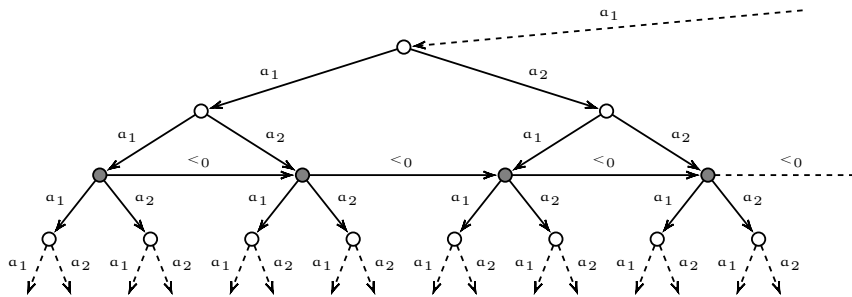
Fig. 3.22. The 2-refinable TULS
