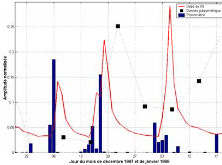
Figure 20 : Superposition des débits (normalisés) de l'III (en rouge), des précipitations efficaces (en bleu) et d'une chronique piézométrique (carrés noirs).
