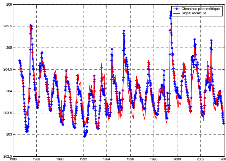
Figure 30 : Comparaison du modèle aux observations
