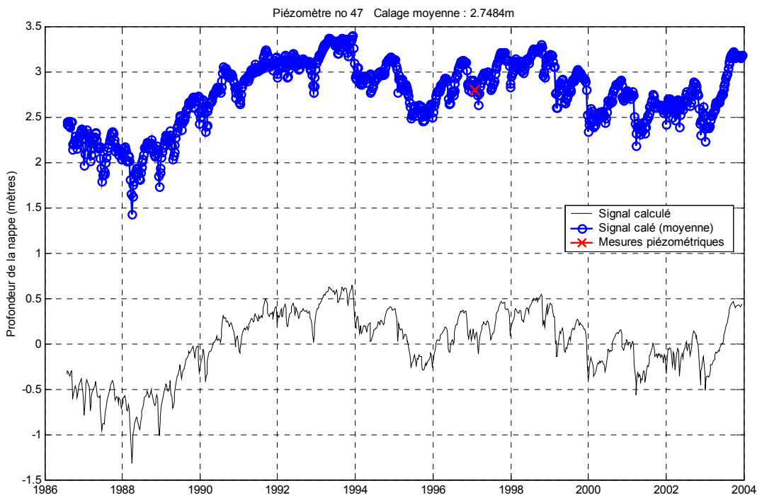
Figure 45 : Superposition d'une mesure piézométrique (en rouge) du signal calculé (en noir) et du signal calé (en bleu) dont la moyenne a été calée
