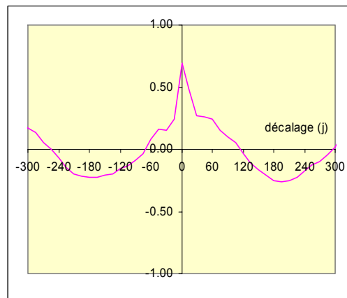
Figure 15 : Corrélogramme croisé Pluie efficace – débit de l'III à Ensisheim. La corrélation observée pour les faibles décalages est comparable à ce qui a été observé avec la Sauer. La courbe de tarissement de l'III décroît pendant une centaine de jours après un événement de pluie.
