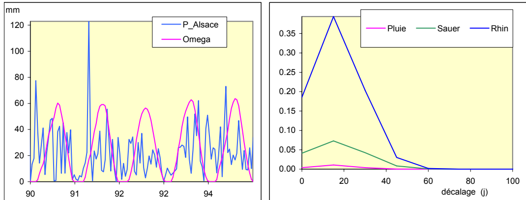
Figure 8 : Calcul de la pluie efficace, hauteur de pluie située au-dessus du seuil \Omega représentant le déficit de la recharge utile des sols et fonctions de transfert. La contribution des 3 composantes aux variations du niveau piézométrique se déduit de l'aire de chacune des 3 fonctions de transfert (respectivement 2%, 17% et 81%).
