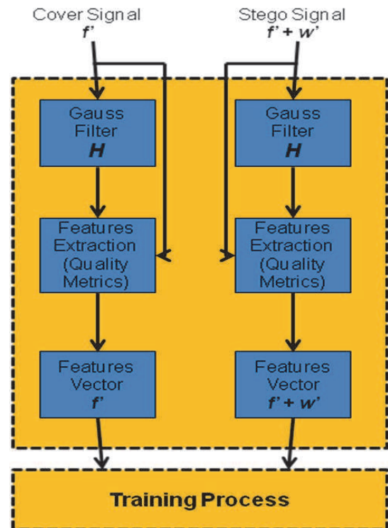
Figura 9 Esquema descriptivo del proceso de esteganalisis
