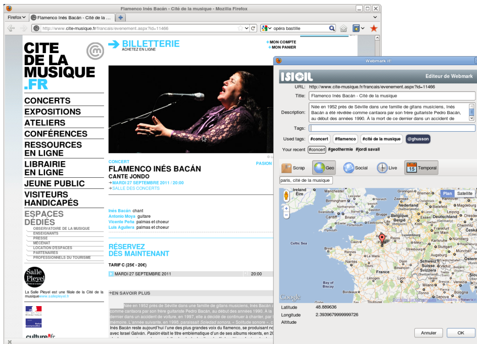
FIG. 4 – Interface Webmarks
