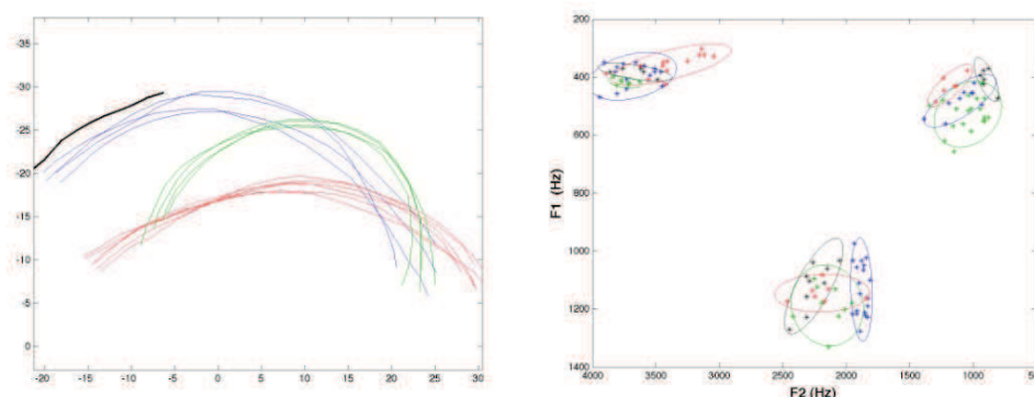
FIGURE 1 – Résultats articulatoires (à gauche) et acoustiques (à droite). À gauche, pour un même sujet : la partie antérieure du palais dur (en noir), quelques exemples de réalisations des voyelles [i] en bleu, [a] en rouge, et de la voyelle [u] en vert. À droite, dans le plan F1-F2, les ellipses de dispersion de chaque sujet (une couleur par sujet) lors de la production de voyelles isolées.
