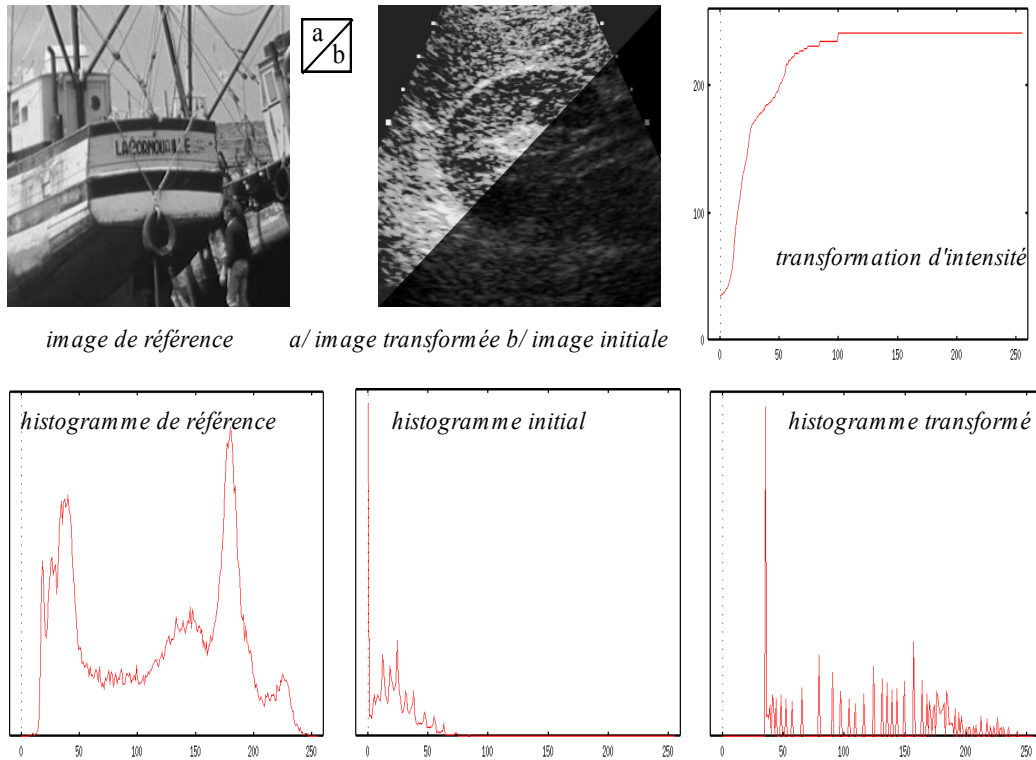
Figure 4.4 : Spécification d'histogramme
