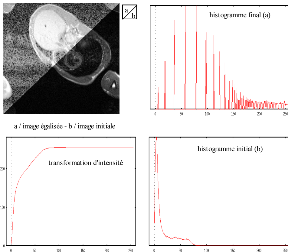
Figure 4.2 : Egalisation d'histogramme
