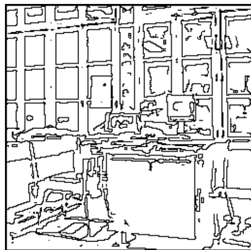
Contours : passages par zéro du laplacien
