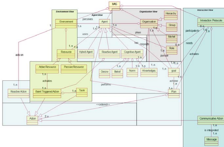
Fig. 8 Agent metamodel (Azaiez, 2007)
