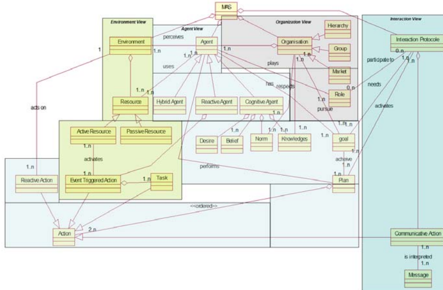
Fig. 8 Agent metamodel (Azaiez, 2007)
