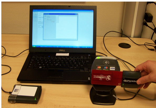
FIGURE 8. Dispositif d'attaque
