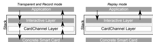
FIGURE 4. Illustration des modes de fonctionnement de la couche Interactive
