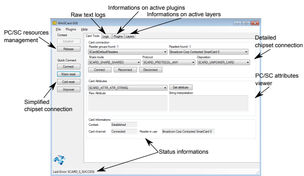
FIGURE 2. Fenêtre principale de l'interface graphique de WinSCard Tools
