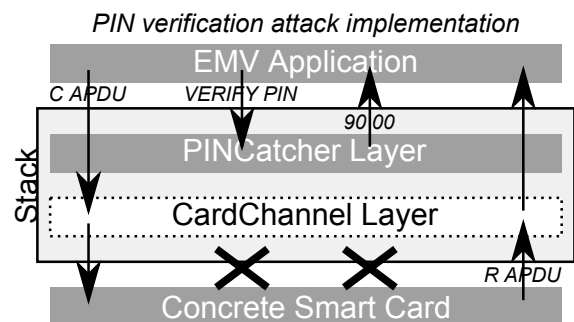
FIGURE 6. Implémentation logicielle de l'attaque sur le code PIN
