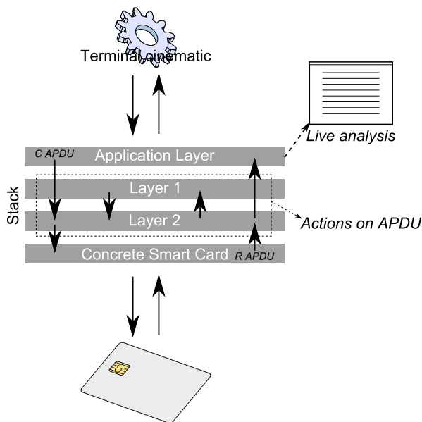
FIGURE 1. Plus value fonctionnelle apportée par l'API de WinSCard Tools
