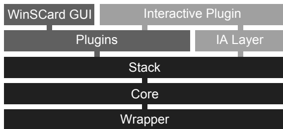
FIGURE 3. Architecture de l'interface graphique
