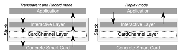
FIGURE 4. Illustration des modes de fonctionnement de la couche Interactive
