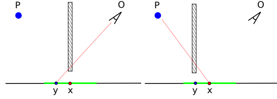
(a) Le photon positionné en y n'est pas visible depuis le point d'observation O (b) La source P du photon n'est pas visible depuis le point d'estimation x
