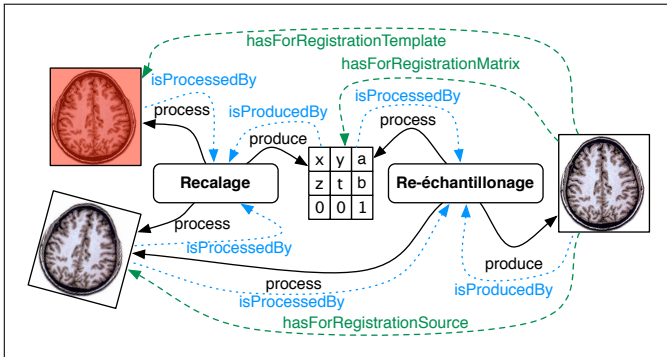
FIGURE 2 – Génération d’annotations sémantiques à l’exécution du flux de calcul.
