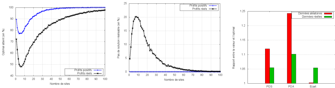
Figure 3: Sur 10 000 tests, nombre de fois où il n'existe pas de solution réalisable au problème MaxSP(pmin), en fonction du nombre de sites.
