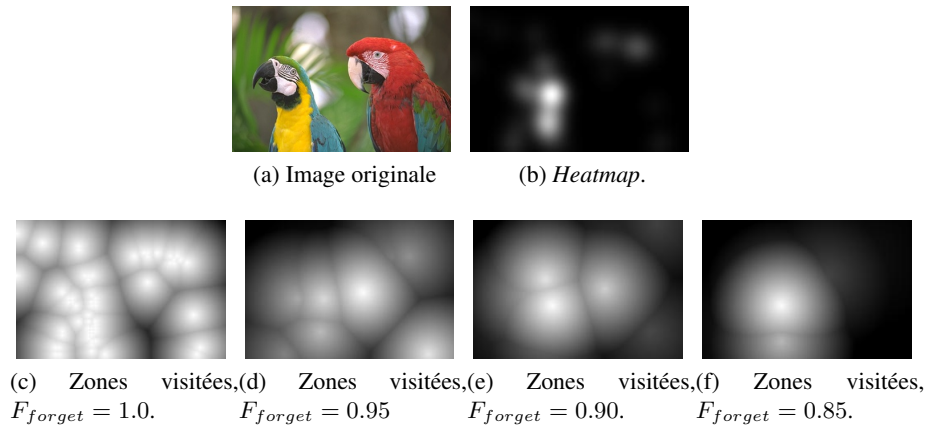
Figure 4: Influence du facteur d'oubli sur la carte des zones visitées après 100 itérations.
