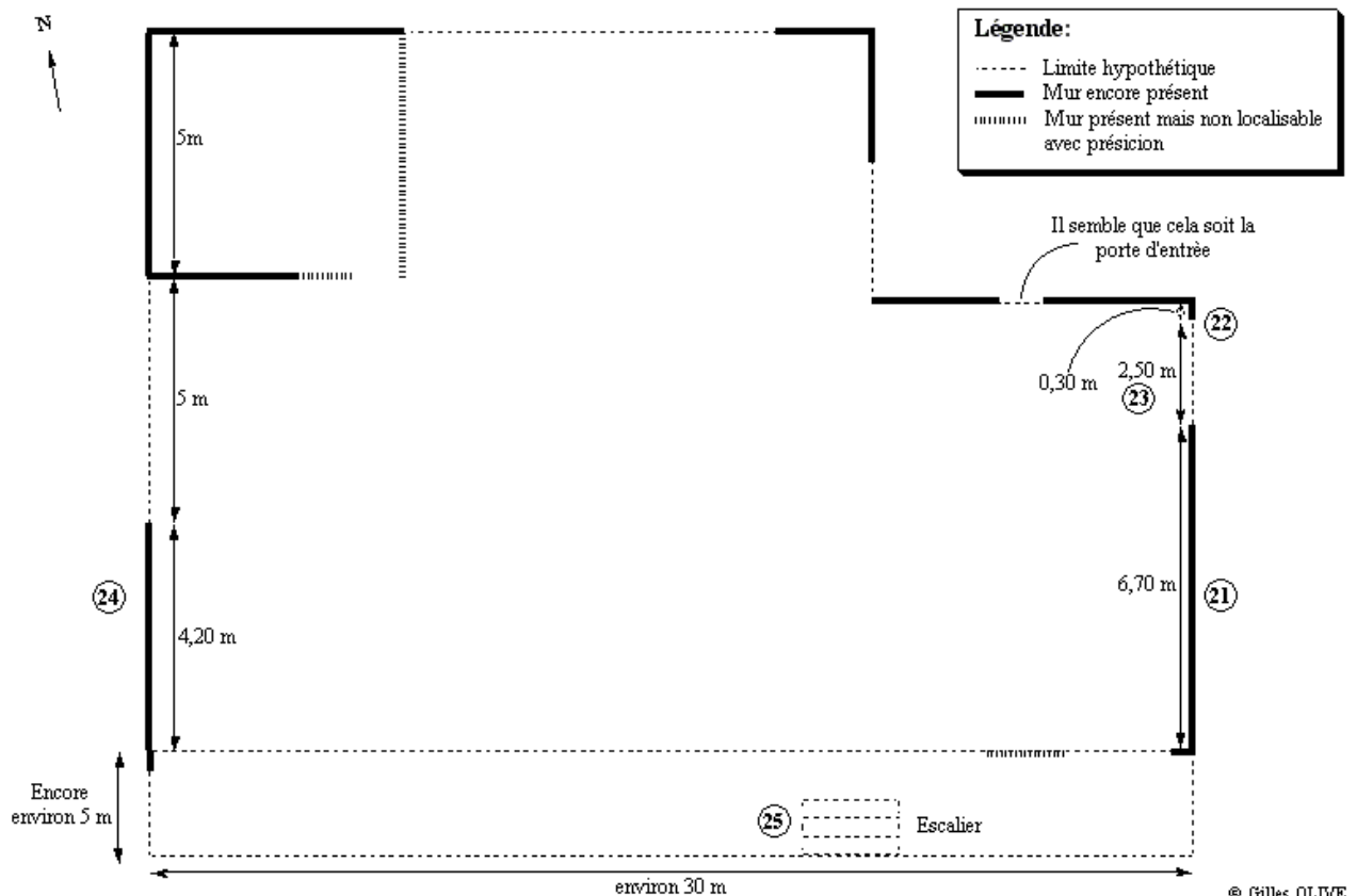
Document 20: Relevé métrique de la soudière. Les chiffres entourés représentent le numéro du document correspondant à la vue. © 2010 Gilles OLIVE.
