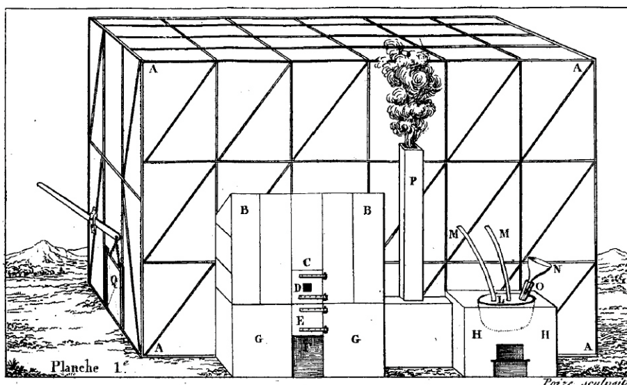
Document 1: Chambre de plomb selon le procédé utilisé à Rouen. Référence 9.
