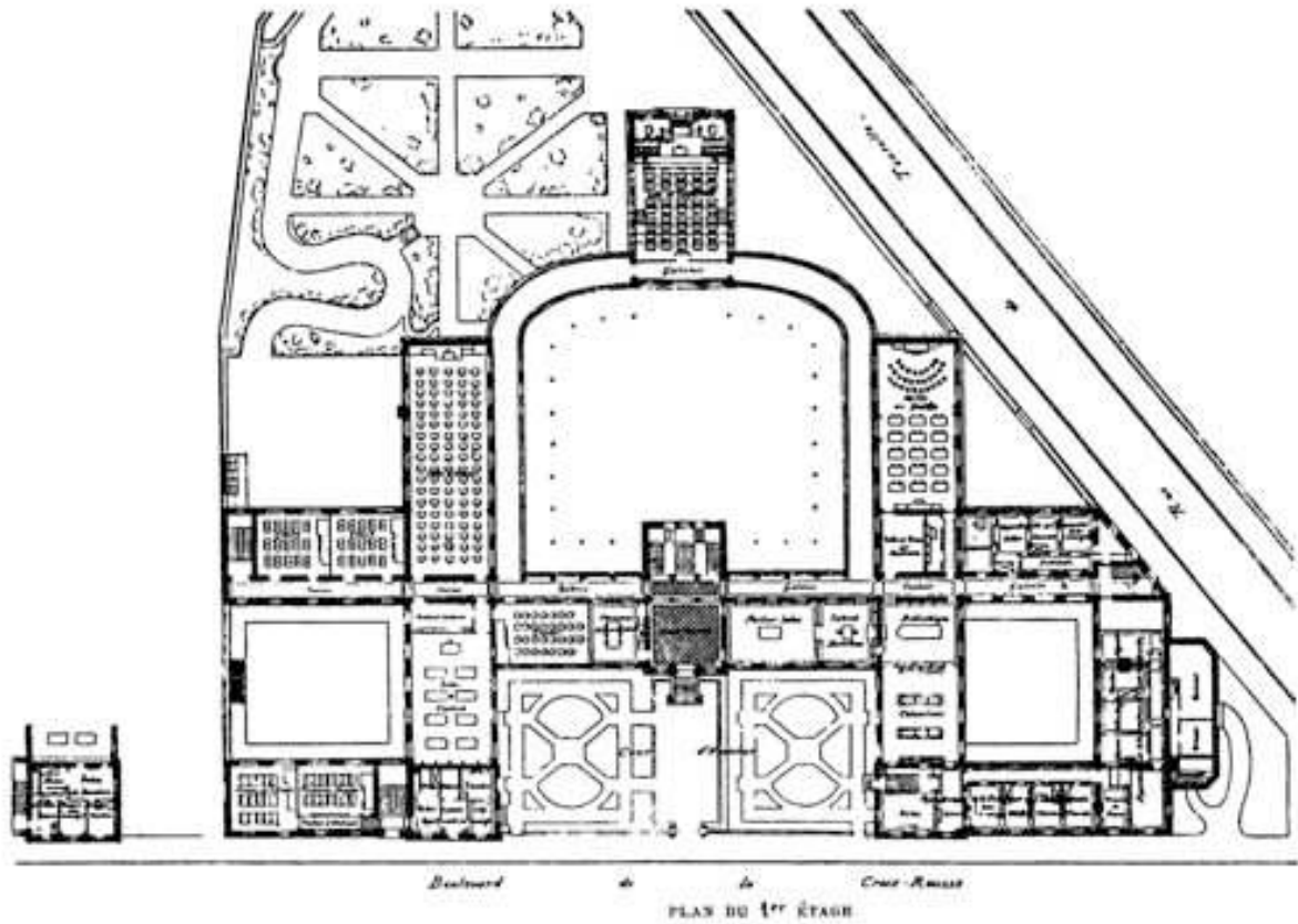
Plan du 1er étage Ph. Geneste, architecte (1879)
