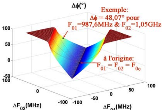
Figure 3. Exemple d'une cartographie du déphasage \Delta\varphi .
