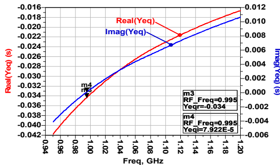
Figure 6. Parties réelle et imaginaire de l'admittance de la partie active de l'oscillateur.
