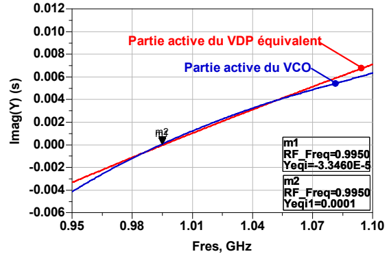
Figure 7. Parties imaginaires des admittances de la partie active du VCO et du VDP.
