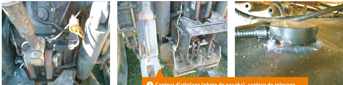
2 Capteur d'attelage (photo de gauche), capteur de relevage (photo centrale), jauge à carburant (photo de droite).
