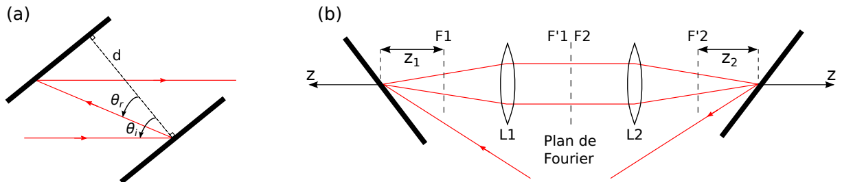
Figure 4. (a) Paire de réseaux induisant une dispersion anormale, (b) utilisation du système afocal afin de changer le signe de la dispersion chromatique.
