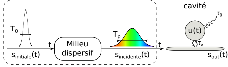
Figure 2. Schéma de principe du dispositif permettant d'introduire une dispersion sur une impulsion limitée par transformée de Fourier.
