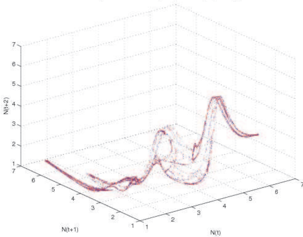
FIGURE 12 – Un comportement complexe : (0,18; 0,30; 8,25) . Les saisons sont continues ( \epsilon_{ete} = 0,1 ). Condition initiale (II). Il semble que T^1 soit mélangeante sur cet attracteur. Dimension fractale estimée : d_f \approx 1,19 .
