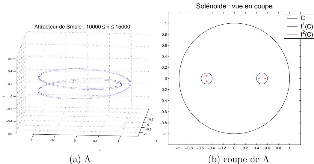
FIGURE 53 – Le solénoïde.
