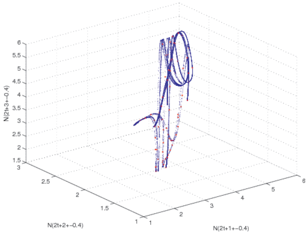
FIGURE 19 – Visualisation de l'attracteur (0,15; 0,30; 8,25) avec une origine des temps \delta = -0,4 .
