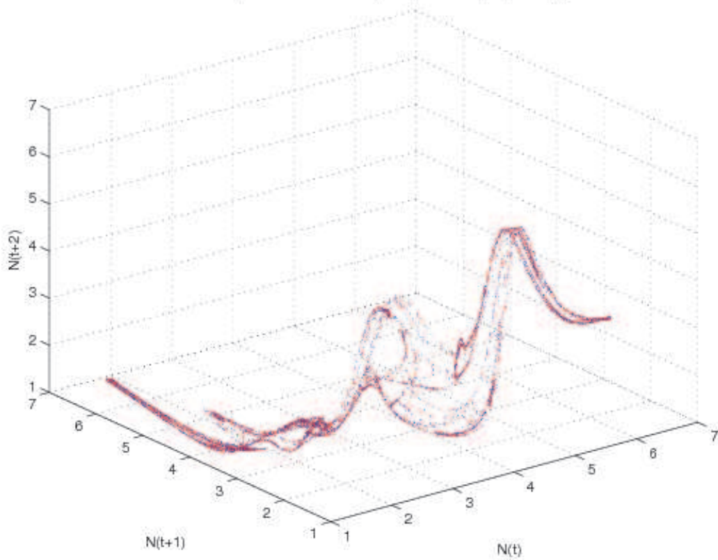
FIGURE 12 – Un comportement complexe : (0,18; 0,30; 8,25) . Les saisons sont continues ( \epsilon_{ete} = 0,1 ). Condition initiale (II). Il semble que T^1 soit mélangante sur cet attracteur. Dimension fractale estimée : d_f \approx 1,19 .
