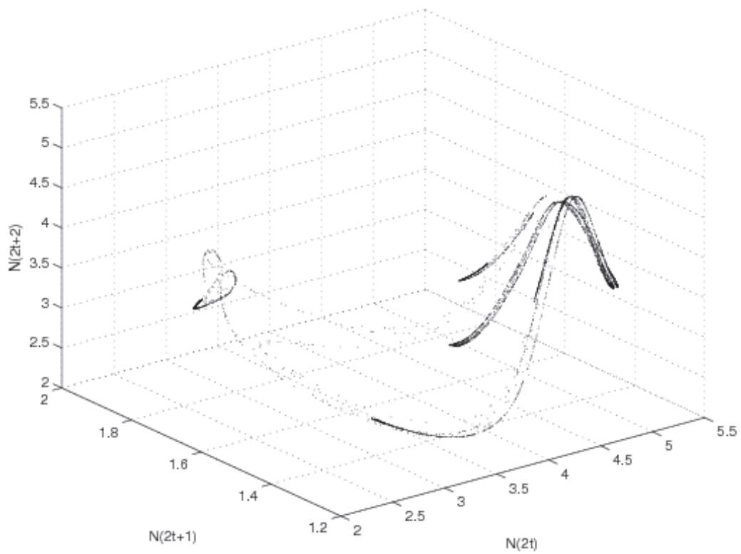
FIGURE 16 – (0,15; 0,30; 8,25) Condition initiale (II). On n’a conservé qu’une composante connexe.
