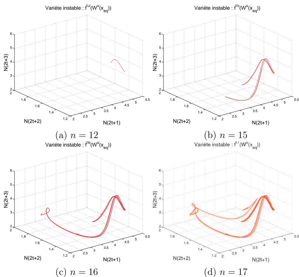
FIGURE 35 – Déploiement de la variété instable à l'équilibre f^n(W^u(x_{eq})) .
