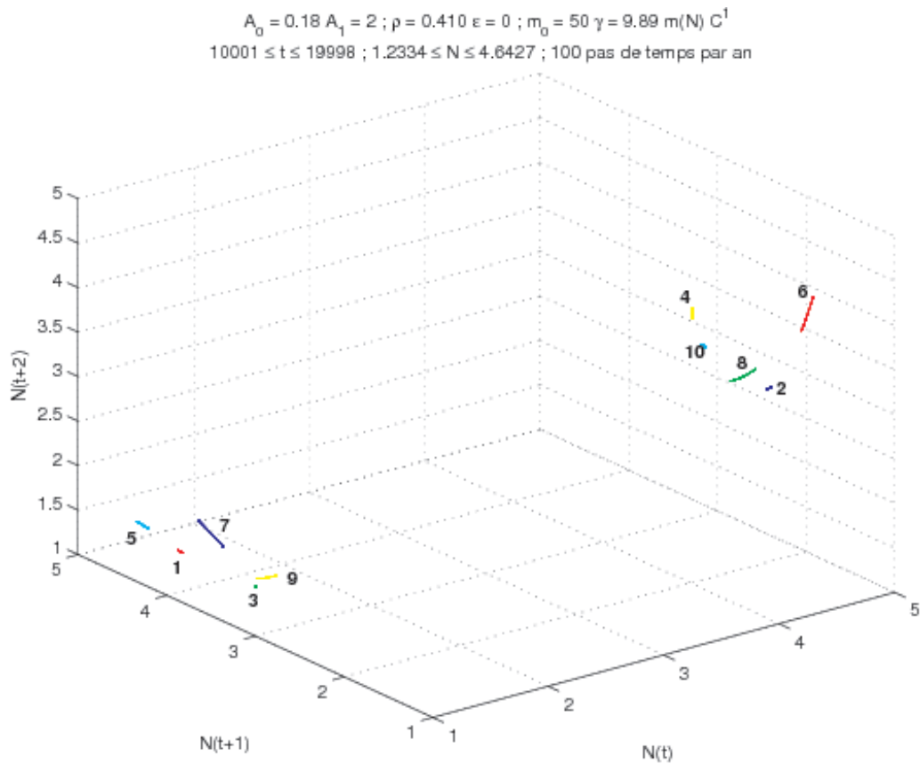
FIGURE 8 – (0,18; 0,41; 9,89). Condition initiale (I). Chacune des composantes est invariante par T^{10} , qui y semble topologiquement mélangeante. La numérotation des composantes correspond aux valeurs de t \bmod 10 . Comme à la figure 7, il y a deux groupes suivant la parité de t . Dimension fractale estimée : d_f \approx 0,92 .
