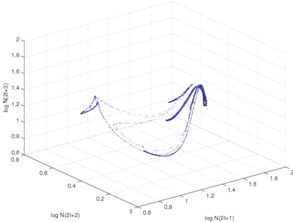
FIGURE 20 – Visualisation de l’attracteur (0,15; 0,30; 8,25) avec une échelle logarithmique.
