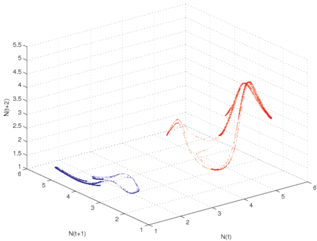
FIGURE 15 – Un comportement complexe : (0,15; 0,30; 8,25) . Condition initiale (II). Les deux composantes sont invariantes par T^2 , qui semble topologiquement mélangeante sur chacune.
