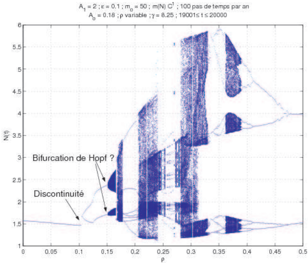
FIGURE 11 – Diagramme de bifurcation (0,18; \rho; 8,25)_{0 \leq \rho \leq 0,5} . Les saisons sont continues ( \varepsilon_{ete} = 0,1 ). Condition initiale (II).
