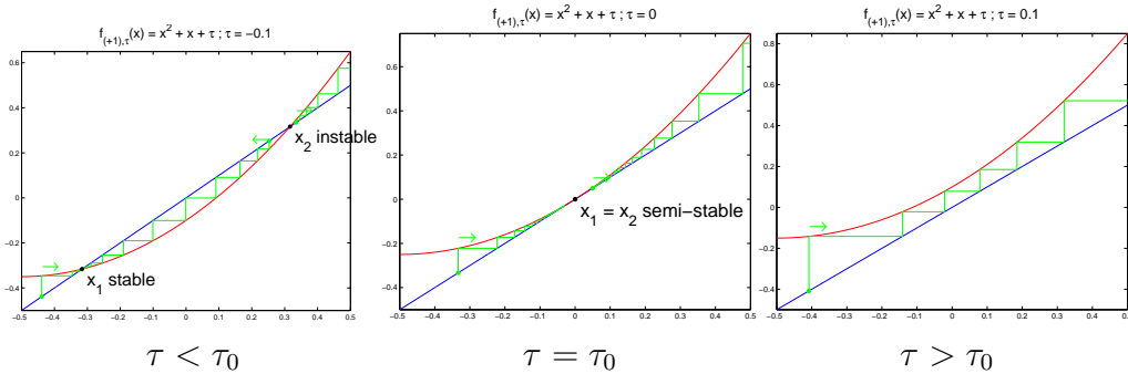
FIGURE 55 – Bifurcation de la famille f_{(+1),\tau}(x) .
