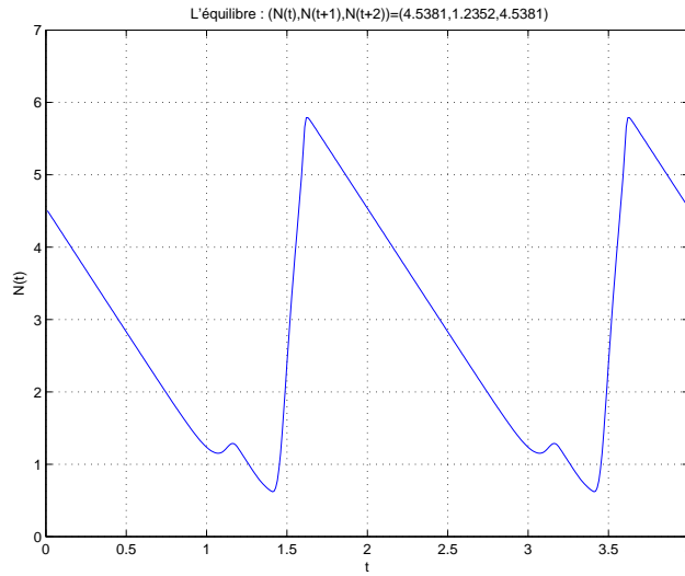
FIGURE 30 – L'équilibre : temps continu.
