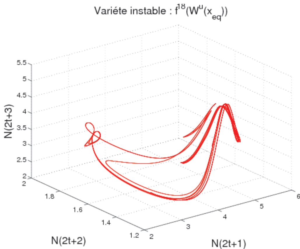
FIGURE 34 – Variété instable.
