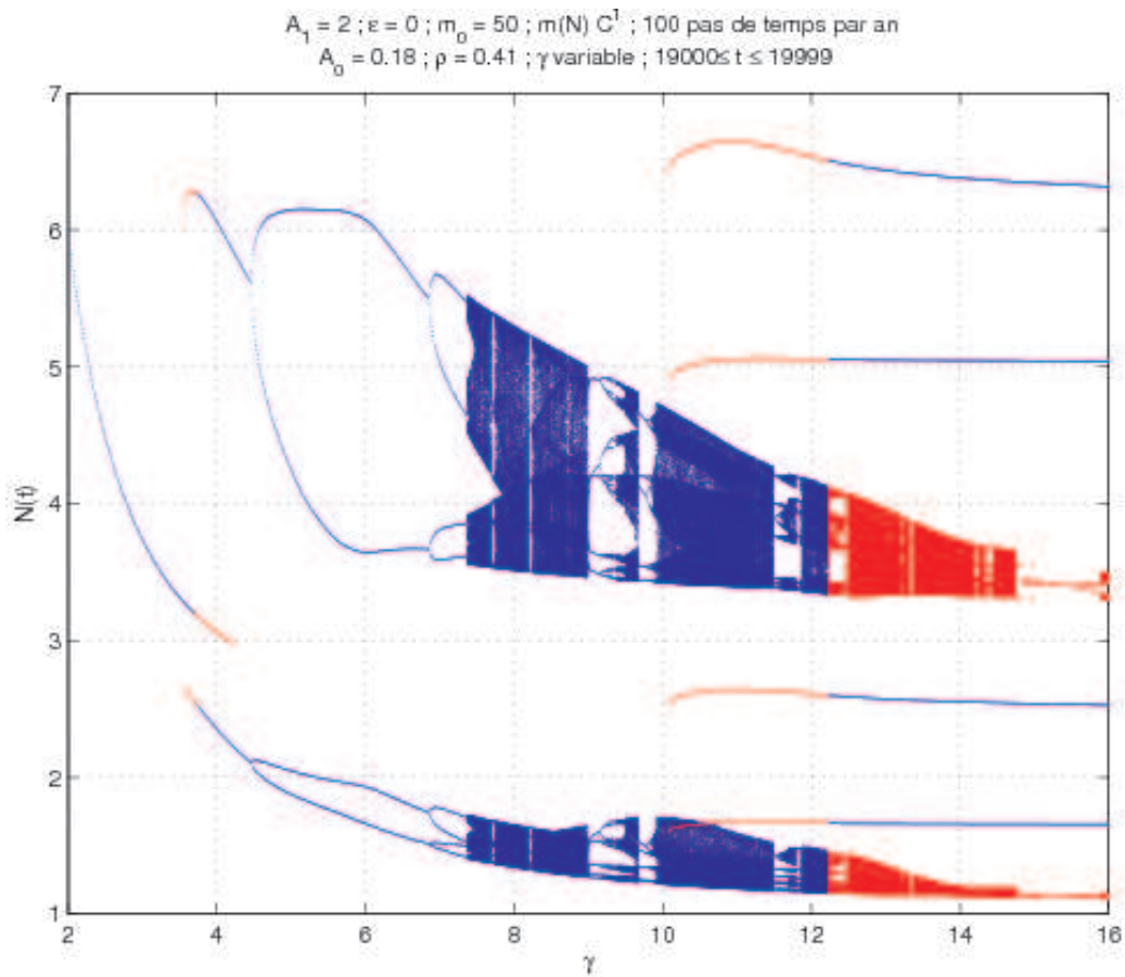
FIGURE 5 – Diagramme de bifurcation (0,18; 0,41; \gamma)_{2 \leq \gamma \leq 16} . Pour certaines valeurs de \gamma , plusieurs attracteurs coexistent. On les a obtenus en utilisant la condition (I) (en bleu) et en prolongeant aussi loin que possible (en rouge) certaines branches interrompues dans le diagramme bleu. Noter que les saisons sont discontinues ( \epsilon_{ete} = 0 ).
