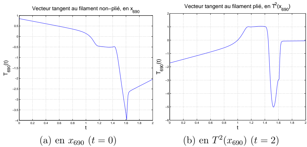
FIGURE 40 – Vecteurs tangents au filament.
