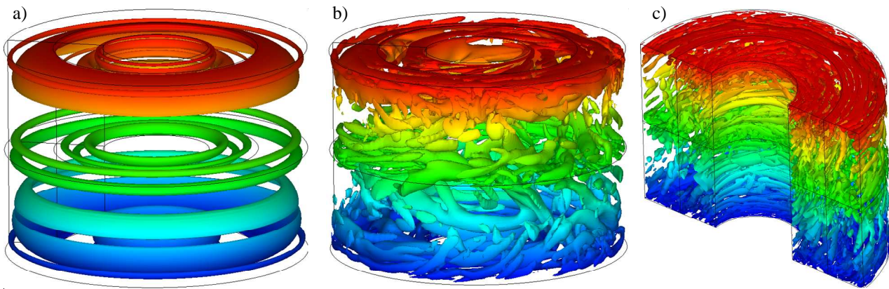
FIG. 2 – Iso-surfaces du critère Q (colorées par la position axiale z ) obtenues par DNS pour a) Re = 3 \times 10^3 , iso-Q = 5 , b) Re = 10^4 , iso-Q = 50 , c) Re = 5 \times 10^4 , iso-Q = 5000 .
