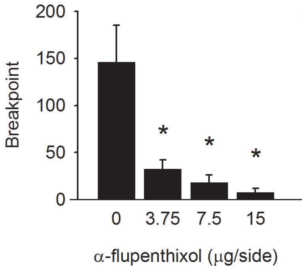
A NAcc shell
