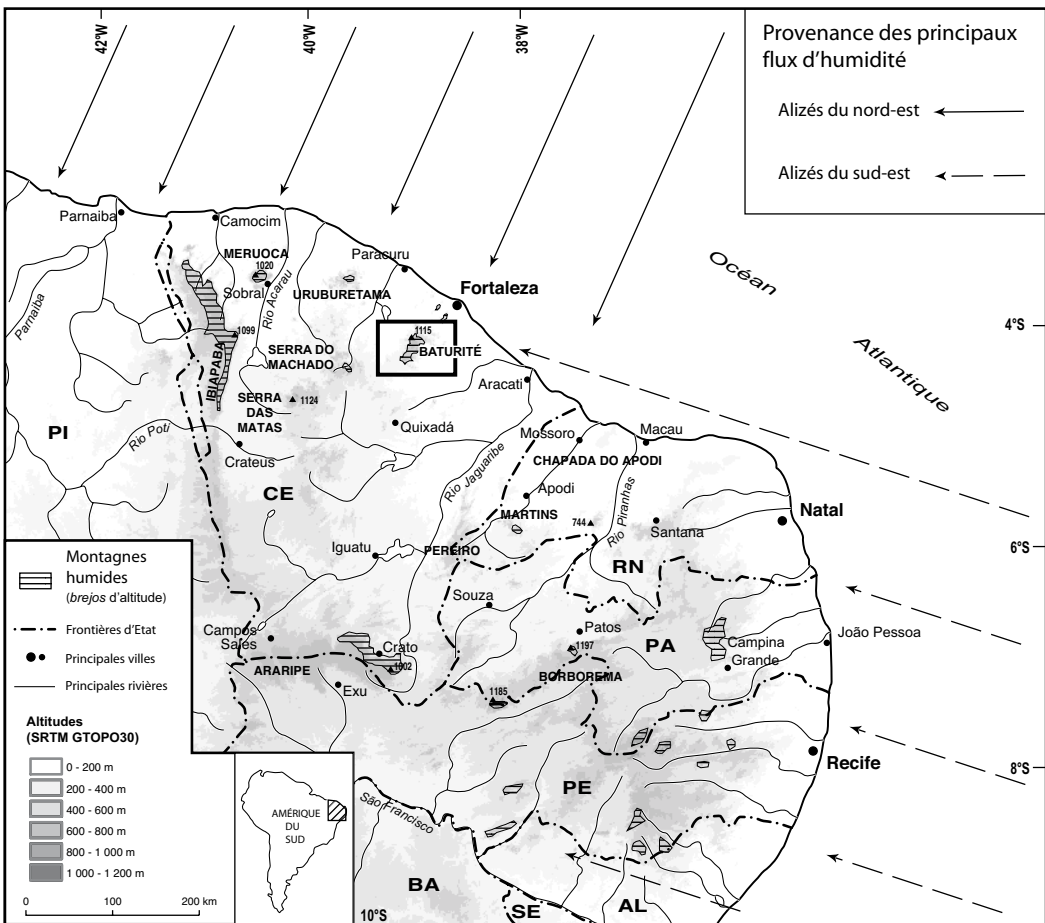
Figure 1 : Répartition des montagnes humides (ou Brejos d'altitude) du Nordeste brésilien et relations avec les principaux flux atmosphériques d'humidité AL : Alagoas; BA : Bahia; CE : Ceará; PA : Paraíba; PE, Pernambuco; RN : Rio Grande do Norte; SE : Sergipe. Le rectangle représente la zone détaillée dans la figure 2.
