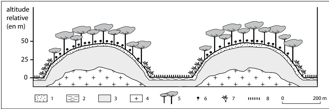
Figure 3 : Modelé multiconvexe forestier et terroirs dans la partie sommitale du massif de Baturité
