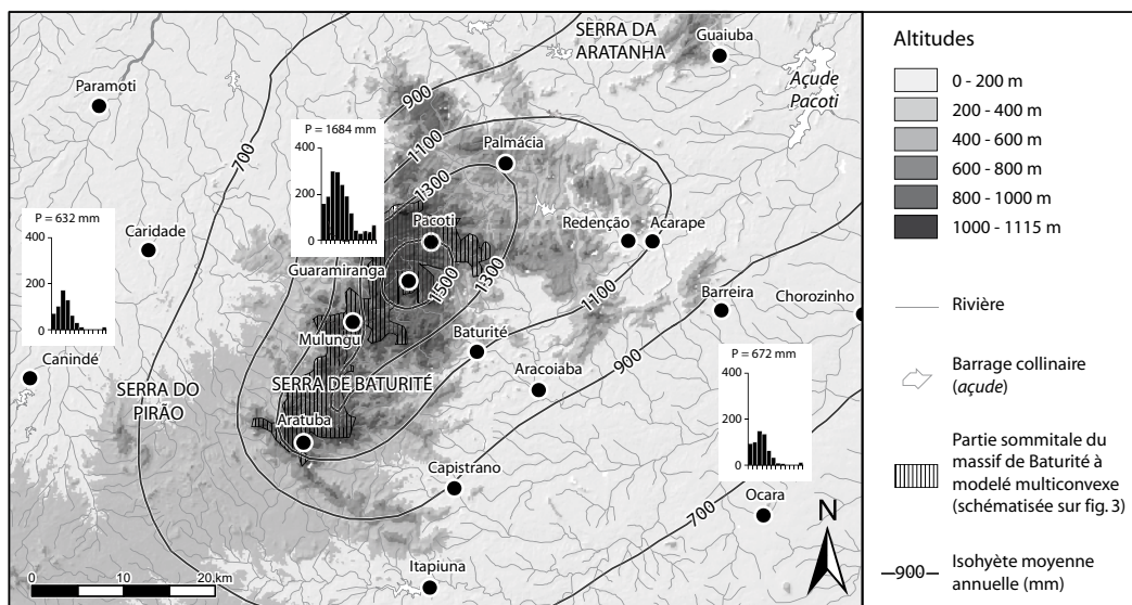
Figure 2 : Le massif de Baturité et son piémont semi-aride : topographie (dérivée du modèle numérique de terrain SRTM 90), pluviosité moyenne annuelle et diagrammes pluviométriques pour trois stations (d'après les données mensuelles de la FUNCEME) (La zone hachurée est schématisée sur la figure 3)
