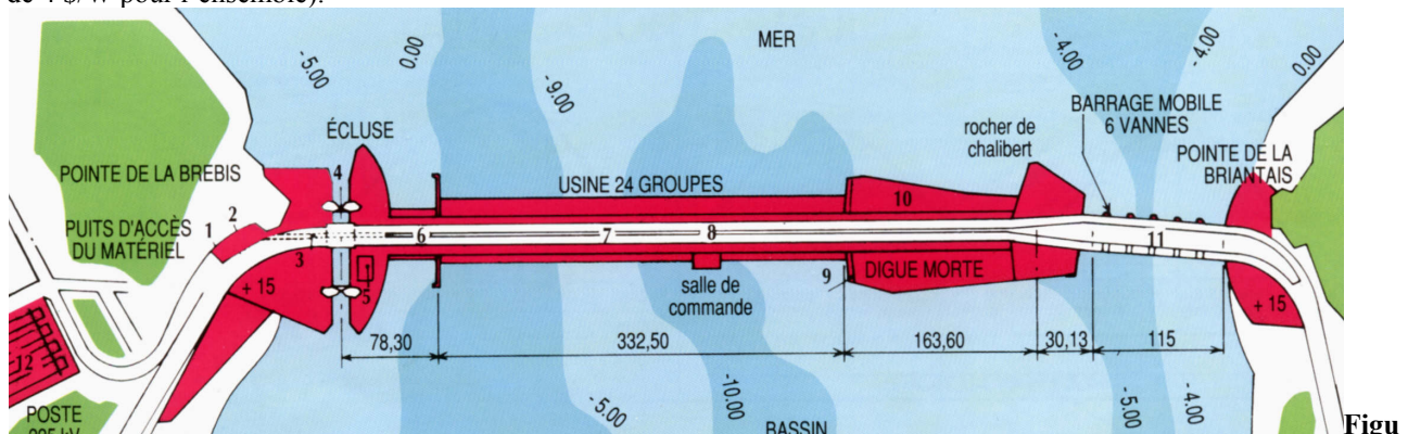
re 7.13. Schéma de l'usine marémotrice de La Rance (240 MW) [ABO 05b]
