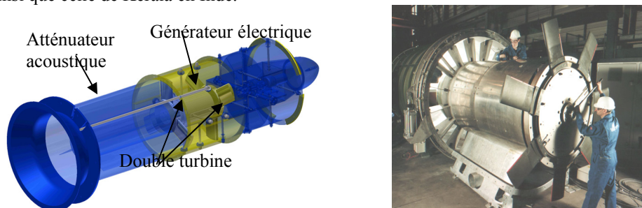
Figure 7.8. Turbogénérateur Wavegen à turbines Wells en cours de montage (groupe de 500 kW), courtesy of Wavegen, [MAC 04].
