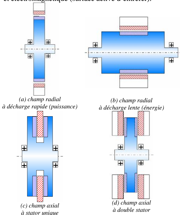
Figure 9. Architectures intégrées de machine électrique possibles pour le stockage inertielle
