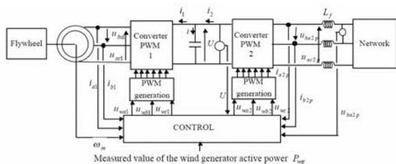
Figure 21b. Schéma de régulation des transferts de puissance du stockage inertiel [18]
